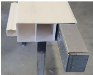
Profilé renforcé par de l'aluminium
