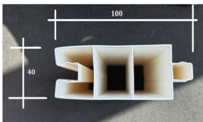
Profilé utilisé pour les murs de la cabine
