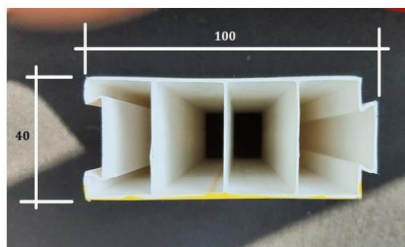
Profilé utilisé pour le toit de la cabine
